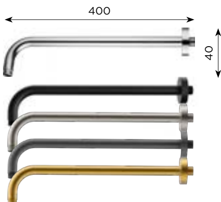
BRAZO ROCIADOR MURAL 400MM
